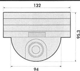
外形寸法
