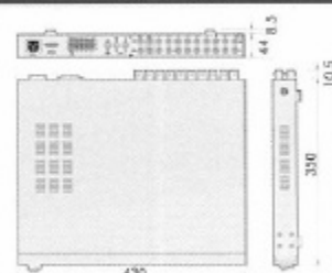
外形寸法
